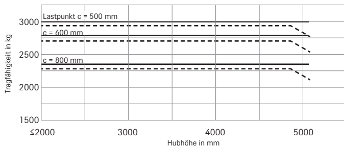
RX 60-30L Teleskop/NiHo-Hubgerüst
